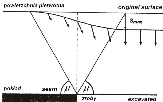
Rys. 1 Ruch punktów na zboczu niecki osiadania [3]
